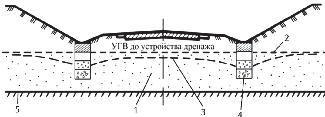
Рисунок 9 – Подкюветный односторонний совершенный дренаж
